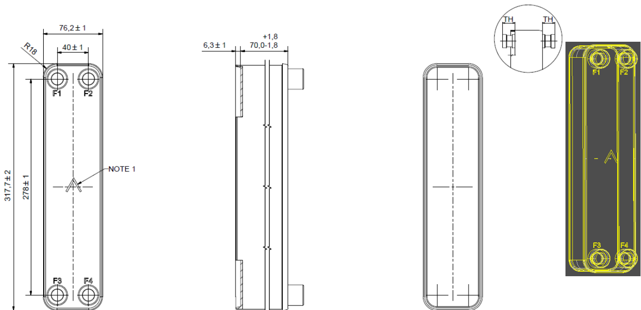
Caracteristicile geometrice ale vaporizatorului
