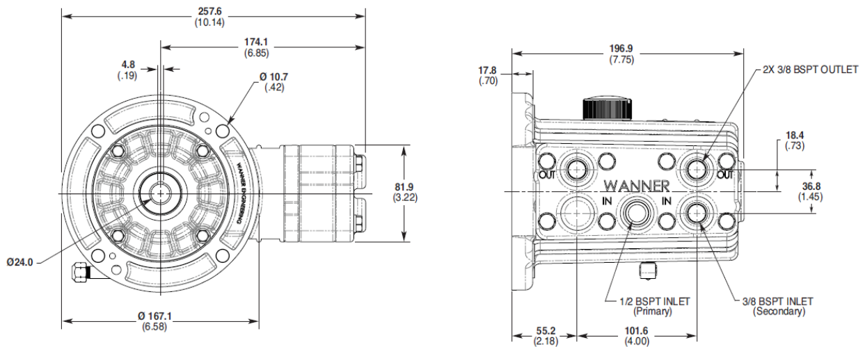
Dimensiunile de gabarit ale pompei fără motorul electric montat (dimensiunile din paranteze sunt în inch)
