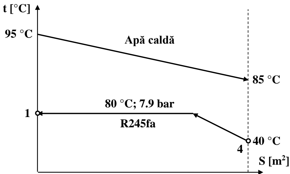
Regimul termic de calcul al vaporizatorului
