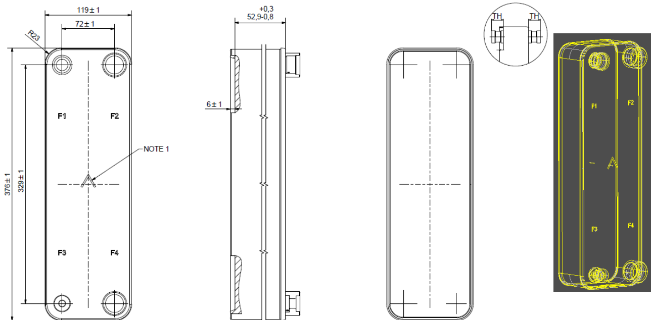
Caracteristicile geometrice ale condensatorului
