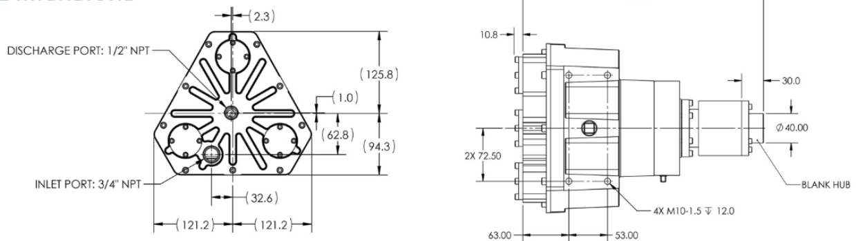
Dimensiunile de gabarit ale detentorului (în mm)
